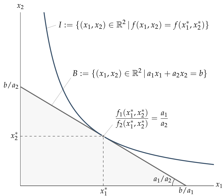
図 19: 最適点 (x_1^*, x_2^*) を通る等高線 I と制約線 B
