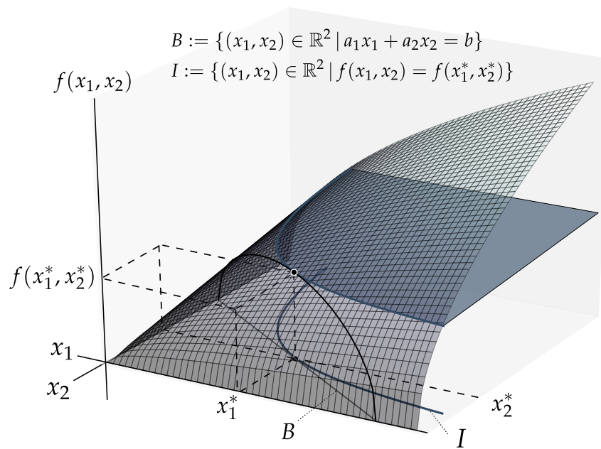
図 18: 2 変数関数 f(x_1, x_2) の制約付最大化
